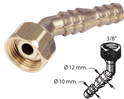
RACCORDO A 45° IN OTTONE PER RUBINETTI
