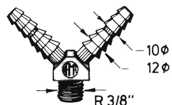
RACCORDO Y IN PLASTICA PER RUBINETTI
