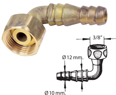
RACCORDO A 90° IN OTTONE PER RUBINETTI
